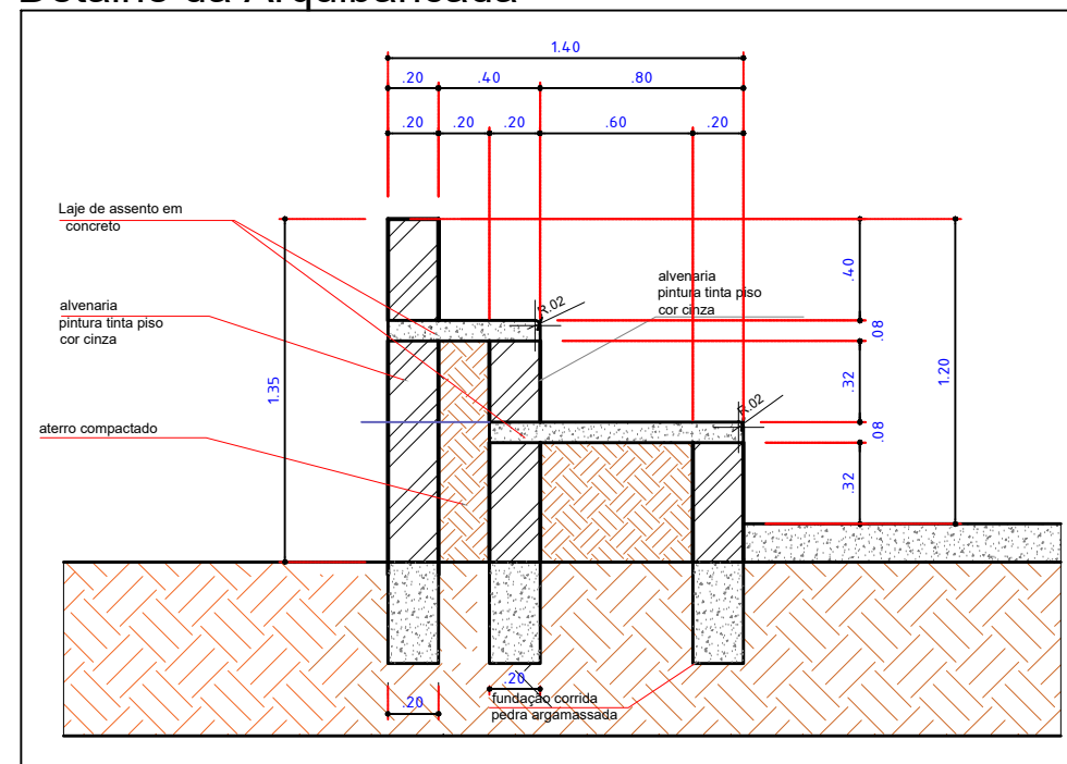
Detalhe da Arquibancada
